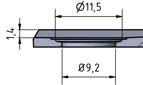
Detalle B
